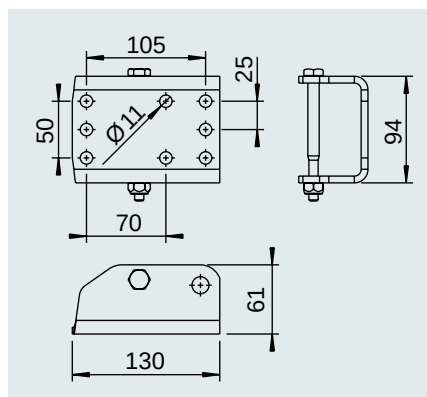
Mittenflansch für Auflaufeinrichtung Profi 3000
