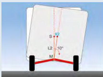
Delta-Schräglenker-Achse
