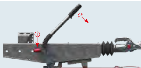
Handbremshebel angezogen = Bremsgestänge gespannt Sperrhebel ① drücken und gleichzeitig Handbremshebel ② absenken
