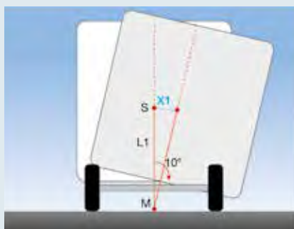
Herkömmliche Achse
