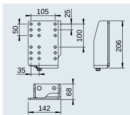
Mittenflansch erhöht für Auflaufeinrichtung Profi 3500
