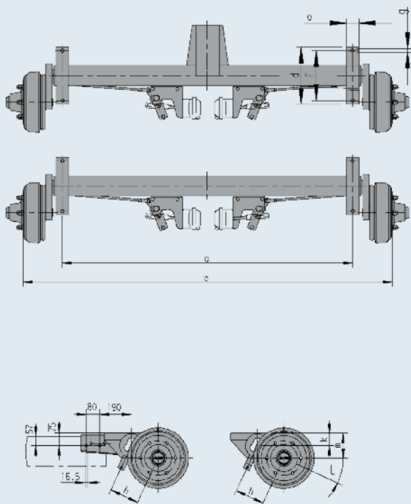
Tandem 3.500 kg Achslast
