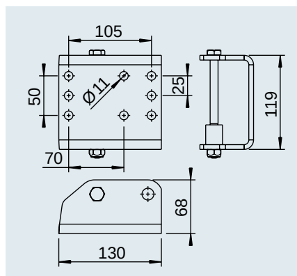
Mittenflansch für Auflaufeinrichtung Profi 3500
