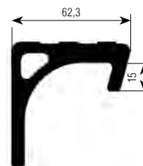
Auflageprofil „A”
