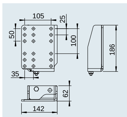
Mittenflansch erhöht für Auflaufeinrichtung Profi 3000
