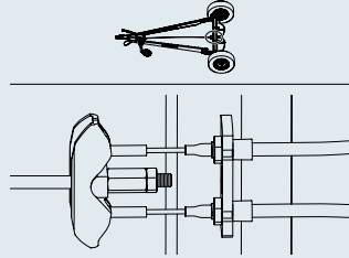
Schnellmontagebowdenzug (1636G, 1637, 2051, 2361)
