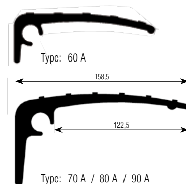
Auflageprofil „B”
