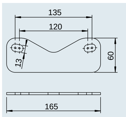
Versteifungsblech für Auflaufeinrichtung Profi 3000/3500
