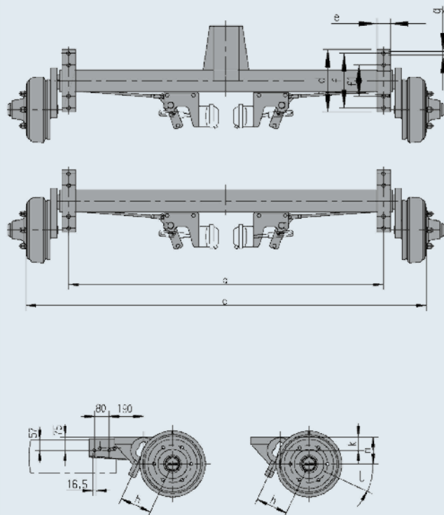
Tandem 5.000 kg Achslast, Tandem 6.000 kg Achslast
